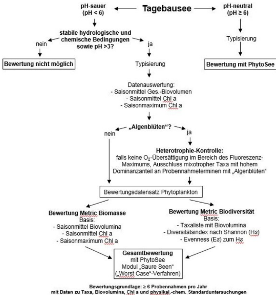
Abb 5: Ablaufschema zur Bewertung des ökologischen Potenzials von Tagebauseen nach LEßMANN & Nixdorf (2009) und LEßMANN et al. (2017)
