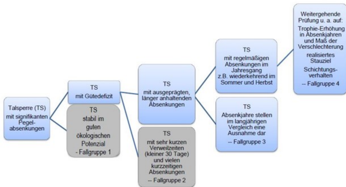
Abb.4: Entscheidungsbaum zur Fallgruppenbildung für die Potenzialbewertung von Talsperren mit Pegelschwankungen. Grau unterlegte Fallgruppe: keine Sonderbehandlung
